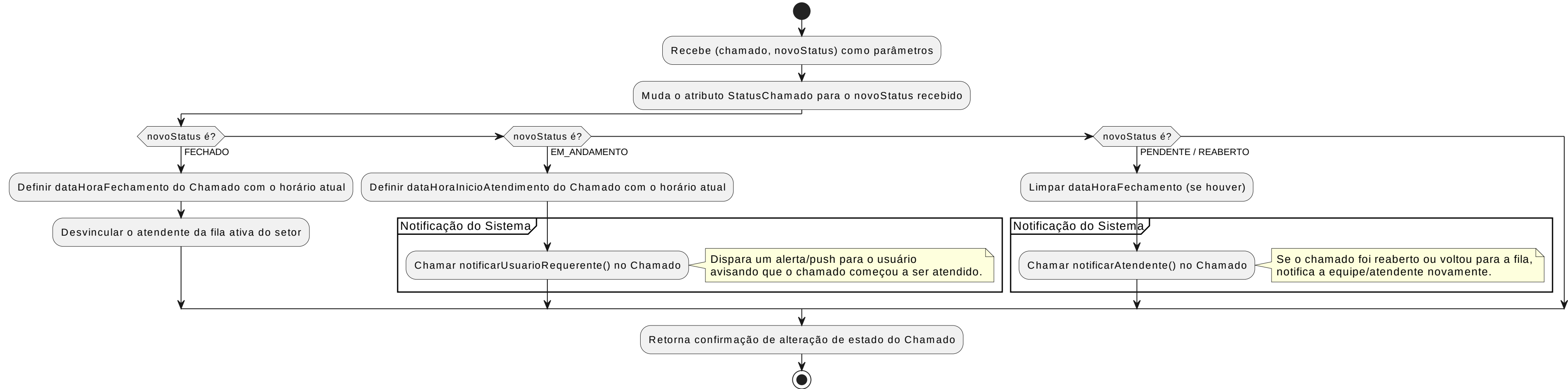
Diagrama de Atividade - Método atualizarStatusChamado()
